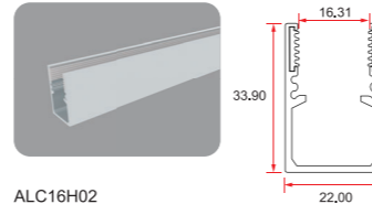
ALC16H02
